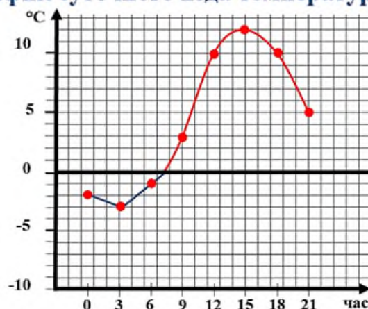
График суточного хода температур воздуха
